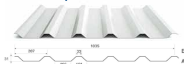
Trapezblech S35/207
