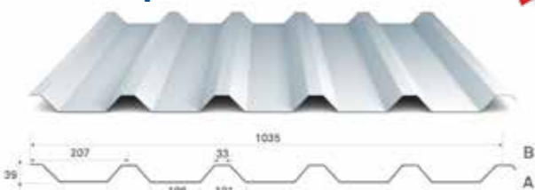
Trapezblech S35/207.PLUS
