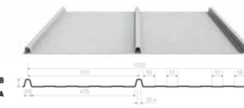
Trapezblech SIEGFALZ S33/510
