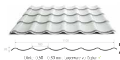
Dachfaltenprofile S26/183
