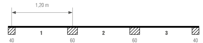
Belastungswerte nach Eurocode 3 (EN 1993-1-3): Profil in Negativlage, Dreifeldträger, Endauflagerbreite 40 mm, Zwischenauflagerbreite 60 mm
